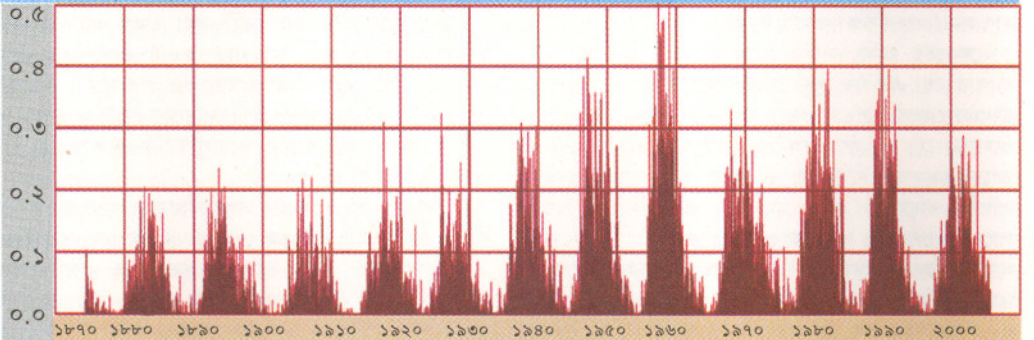
আয়তন (সূর্যের দৃশ্যমান গোলার্ধের আয়তনের শতাংশ)
