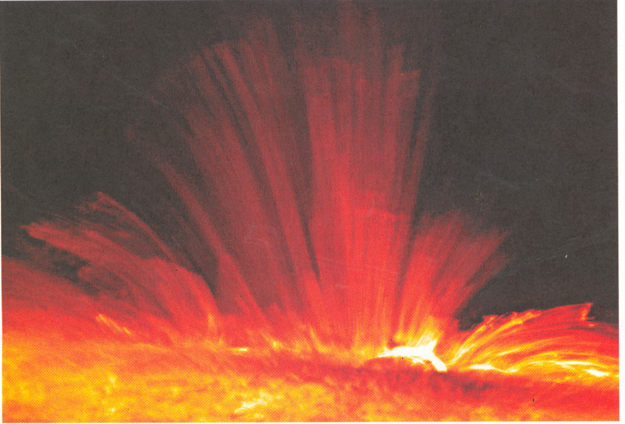
বিষ্ফুর্ত সূর্যের শরীর থেকে বেরচ্ছে সৌরশিখা
