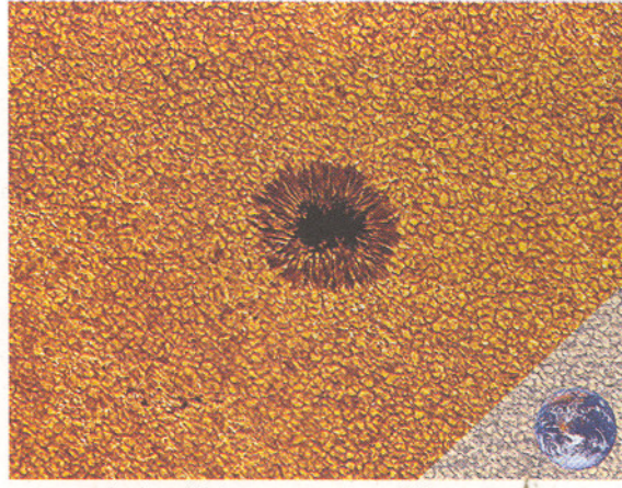
সূর্যপৃষ্ঠে একটি সৌরকলঙ্ক। আয়তনে পৃথিবীর থেকেও বড়
