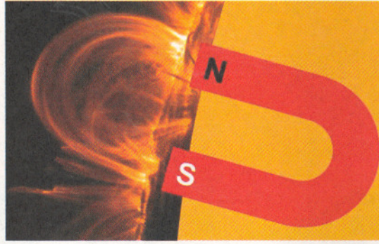
সৌরকলঙ্ক থাকে জোড় বর্ষে, চৌম্বকমেরুর সঙ্গে সংশ্লিষ্ট
